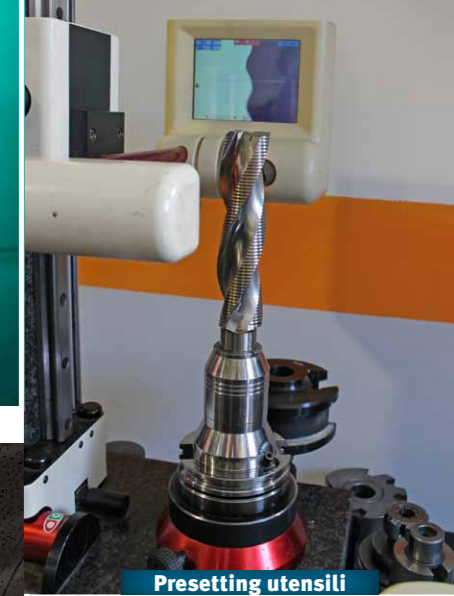
Presetting utensili
